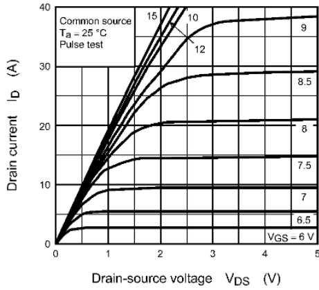
Fig. 8.1 I_D - V_{DS}
