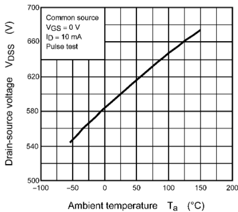
Fig. 8.5 V_{DSS} - T_a
