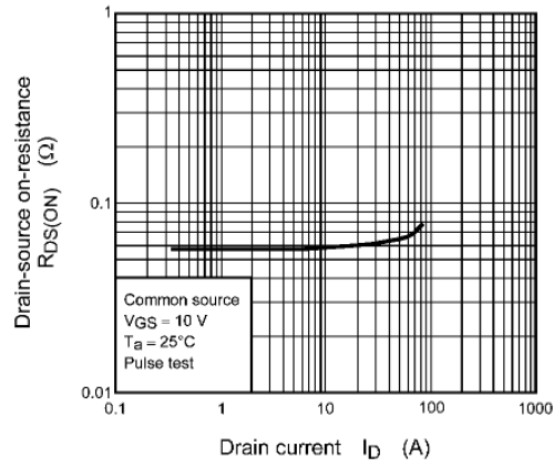
Fig. 8.6 R_{DS(ON)} - I_D
