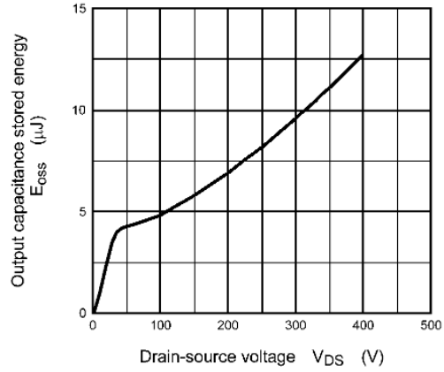
Fig. 8.10 E_{oss} - V_{DS}
